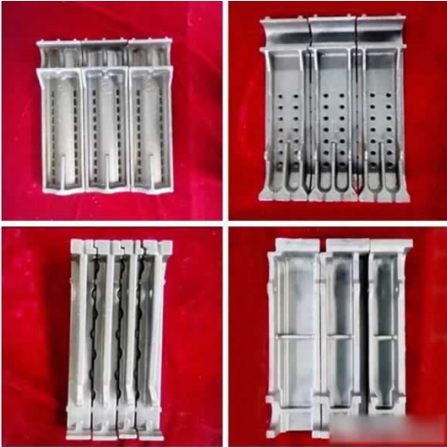
高温合金炉排
