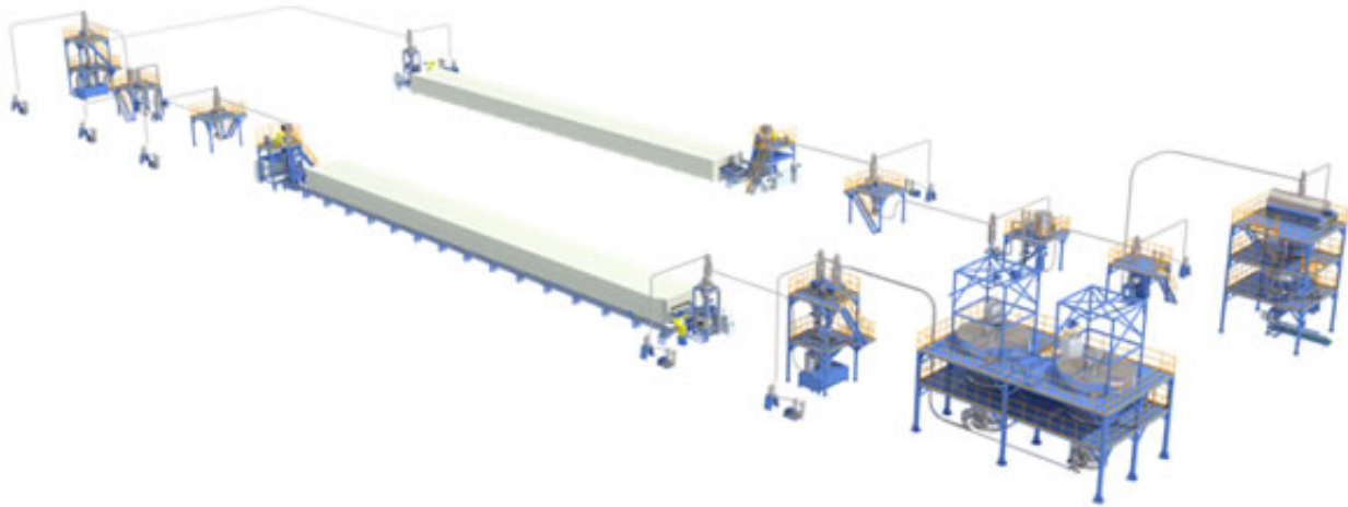
无锡灵鸽-锂电正负极材料制备系统
