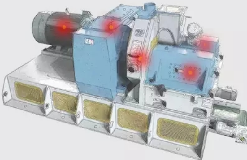
贝尔斯7270颗粒机温度控制系统
