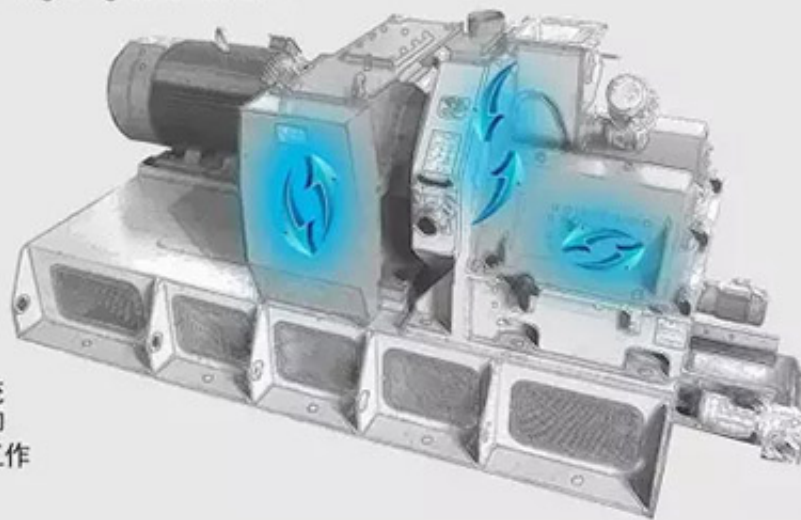
贝斯尔7270颗粒机水循环冷却系统
