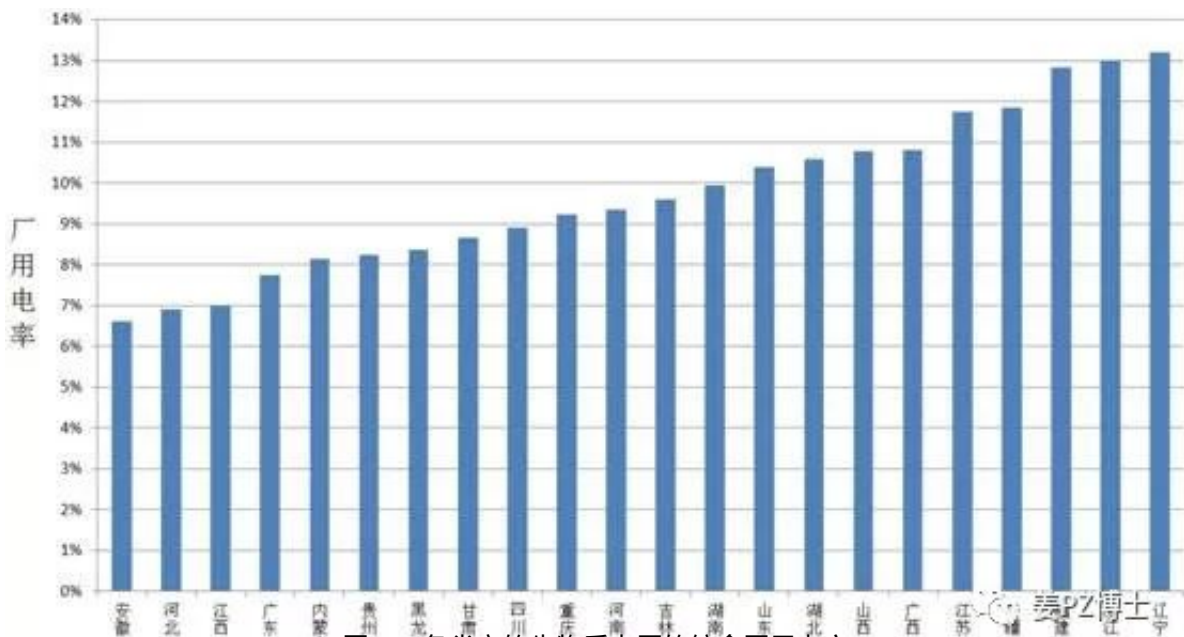
图一、各省市的生物质电厂的综合厂用电率
