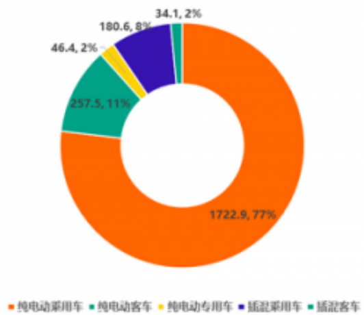
2019年2月动力电池装车量 (单位: MWh)
