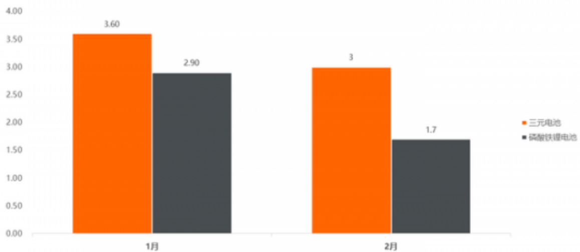
2019年1-2月动力电池产量数据（单位：GWh）
