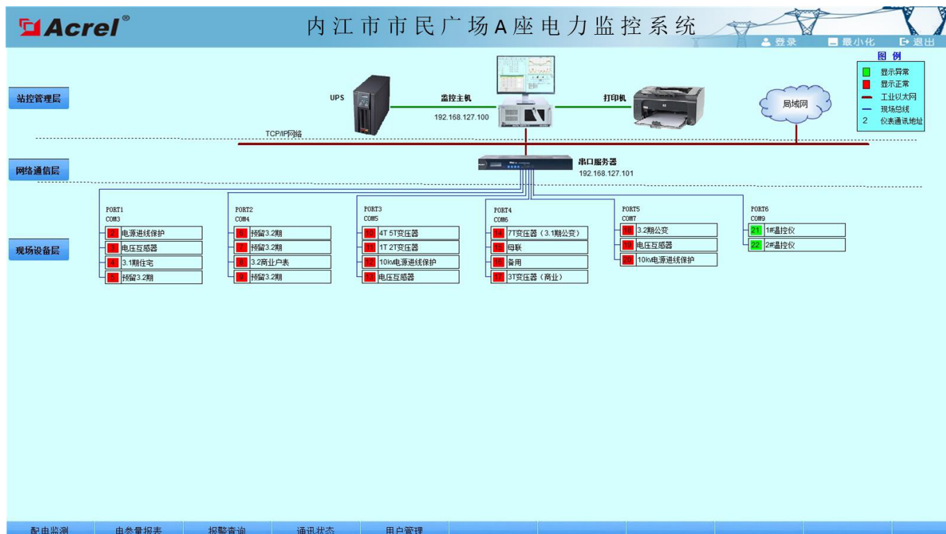
图 (3) 系统通讯结构示意图
