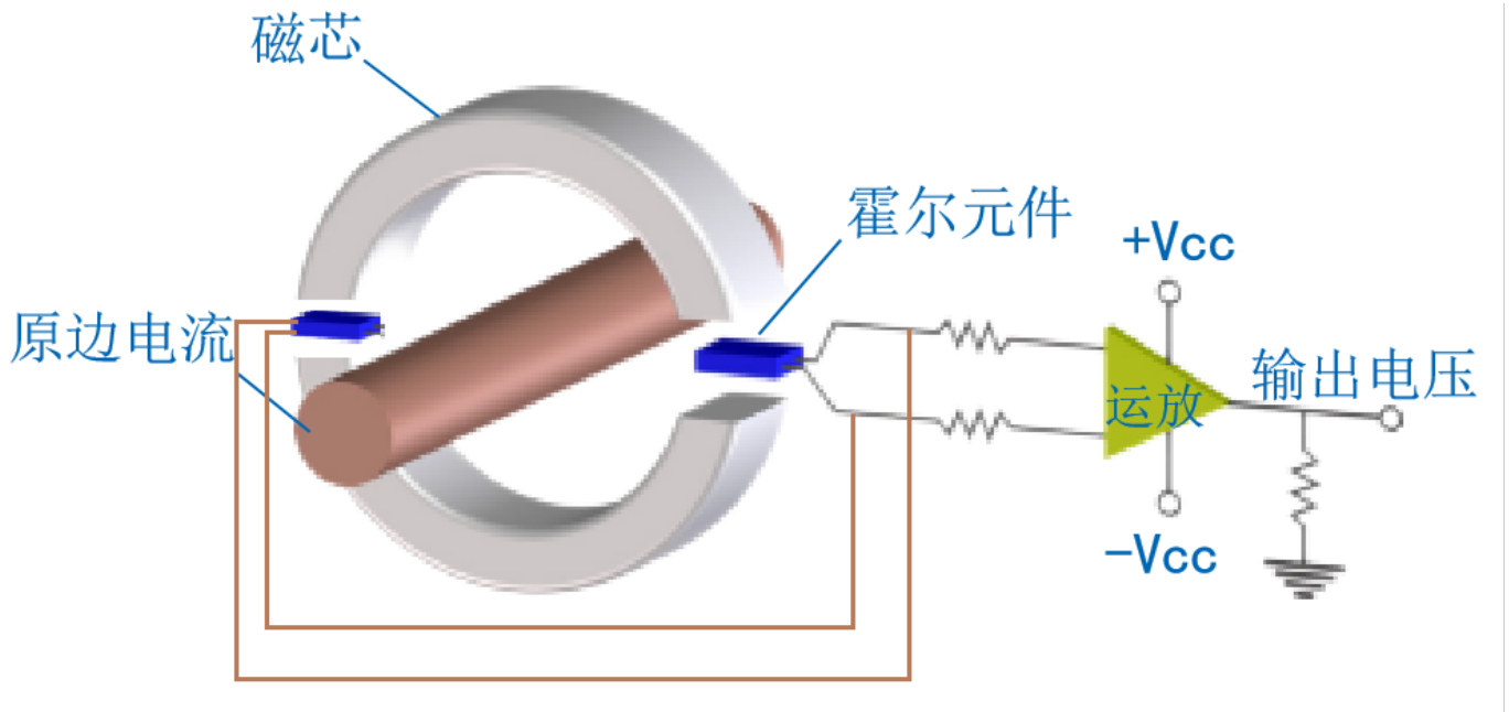
开口式霍尔传感器原理图
