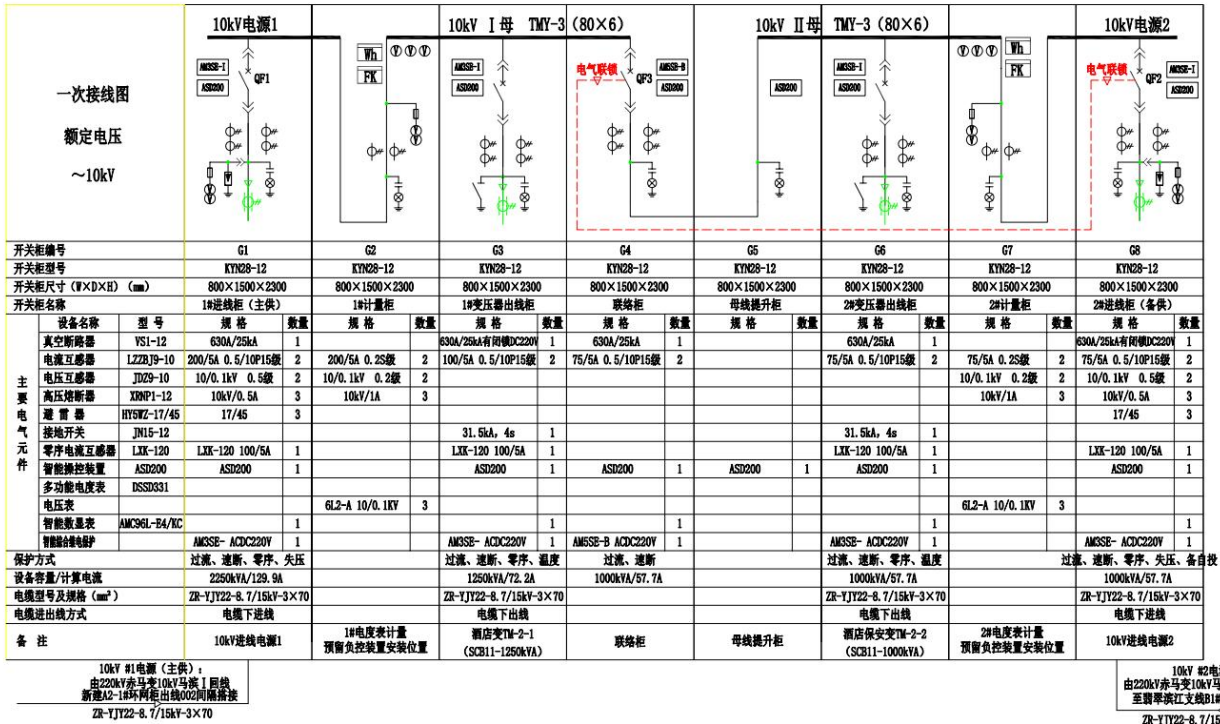
图2 A1-2#酒店配电房上图方案
