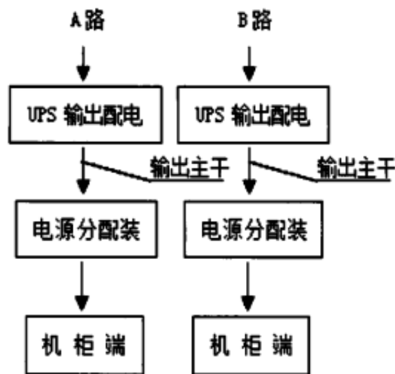
图1 数据中心配电系统拓扑图
