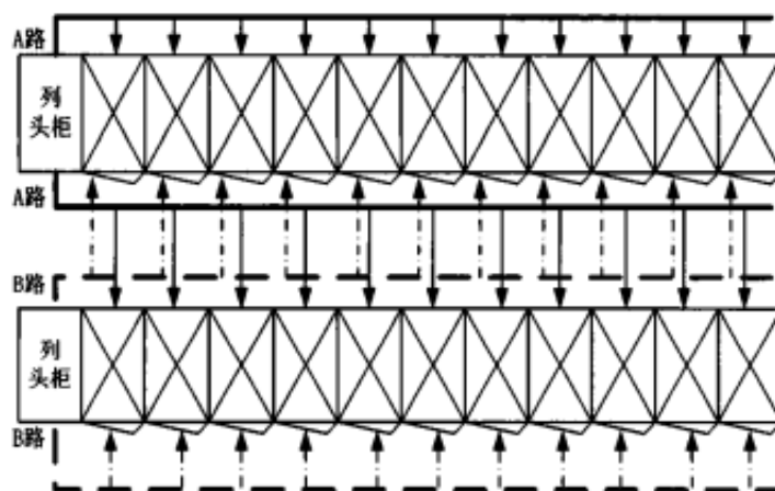
图3 双列头柜供电模式
