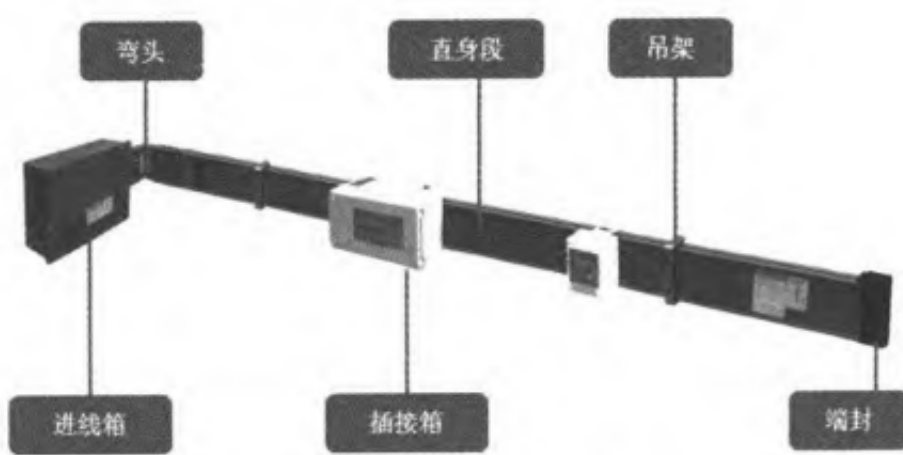
图6 智能母线槽构成图
