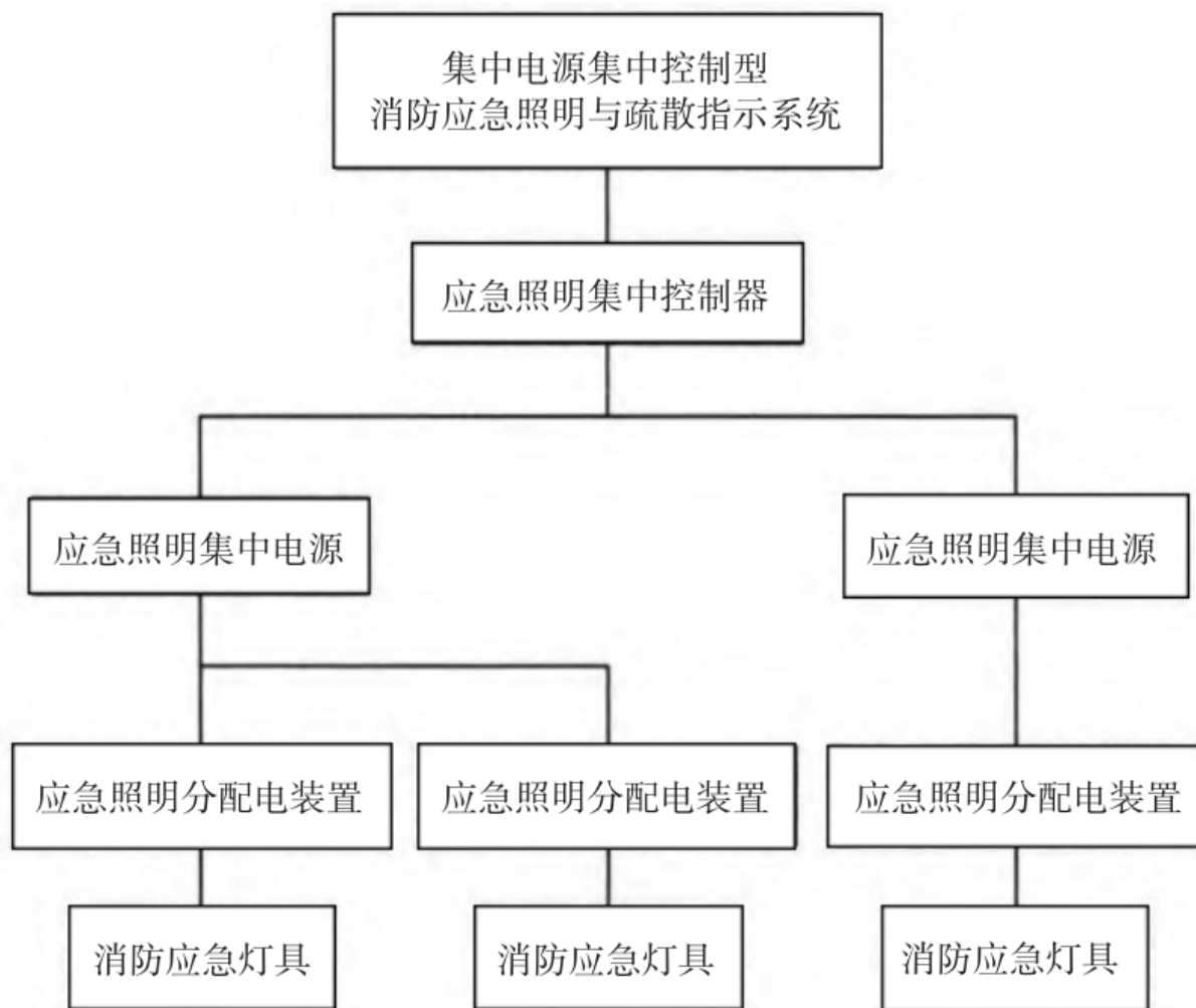
图1 集中电源集中控制型系统
