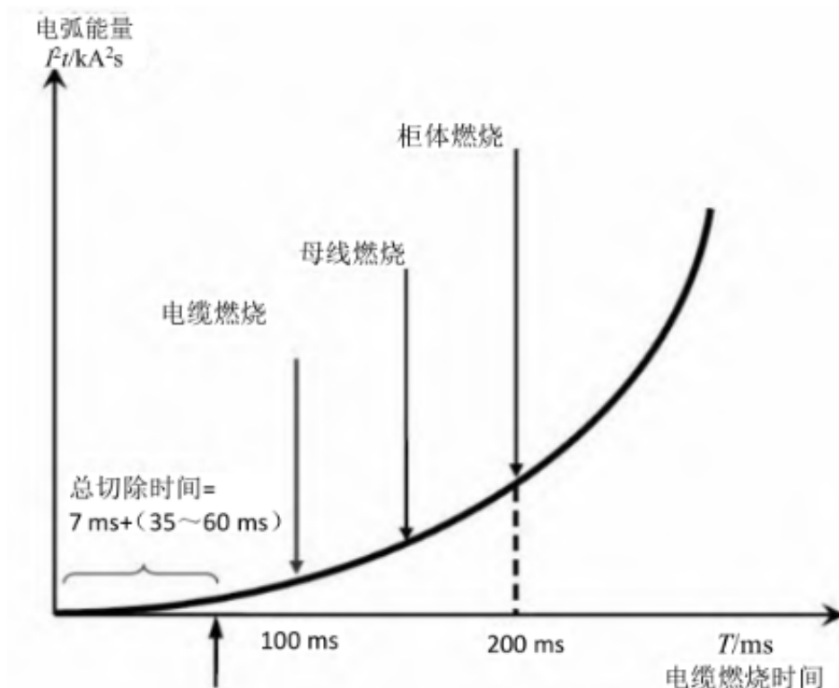
图1电弧光的危害示意图
