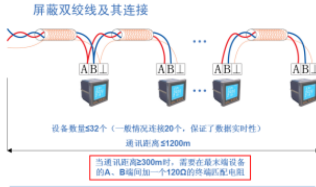
通讯线路连接示意图
