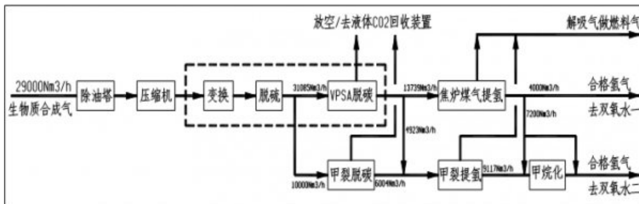
图13 工艺路线图
