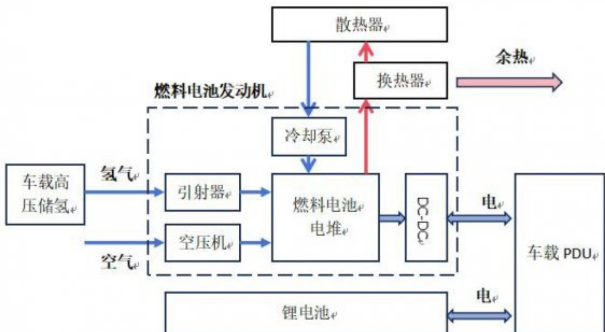
图1 技术原理图
