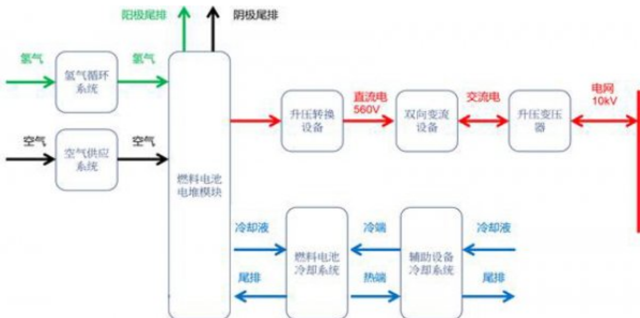
图2 工艺路线图
