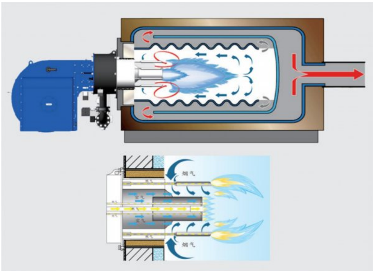
图6 燃烧器结构图
