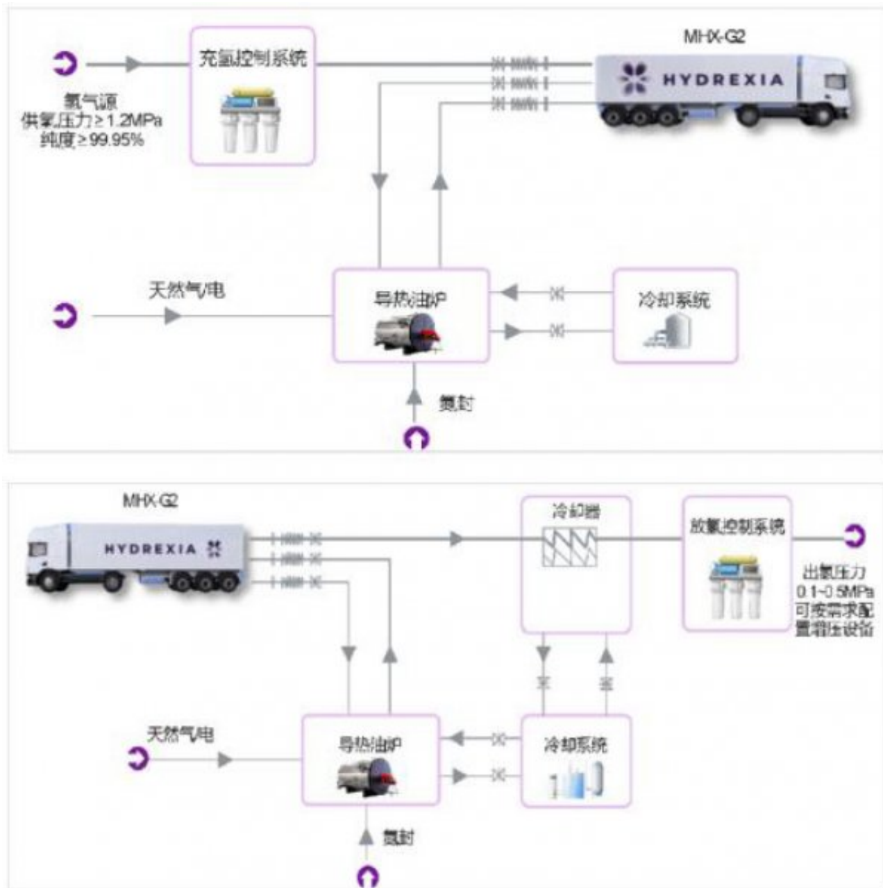
图7 充放氢过程工艺流程图
