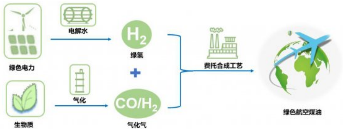
图14 工艺流程图
