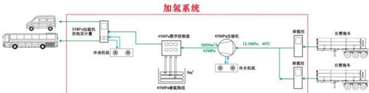
图3 标准加氢站工艺流程图
