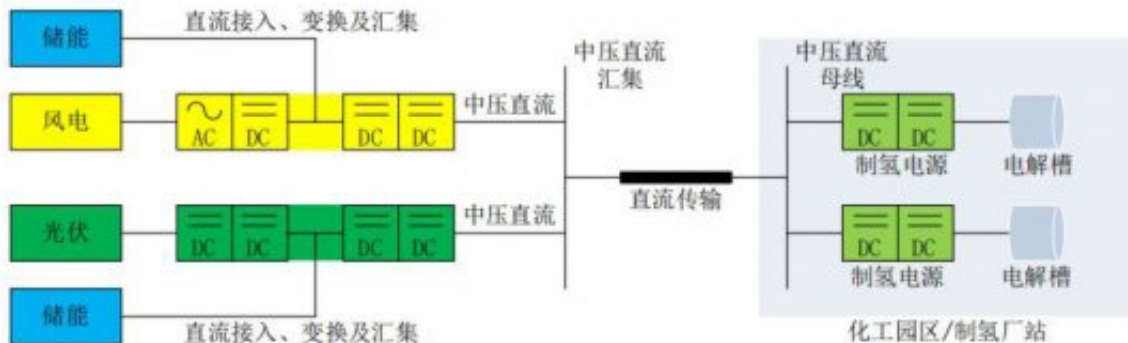
图8 工艺路线图
