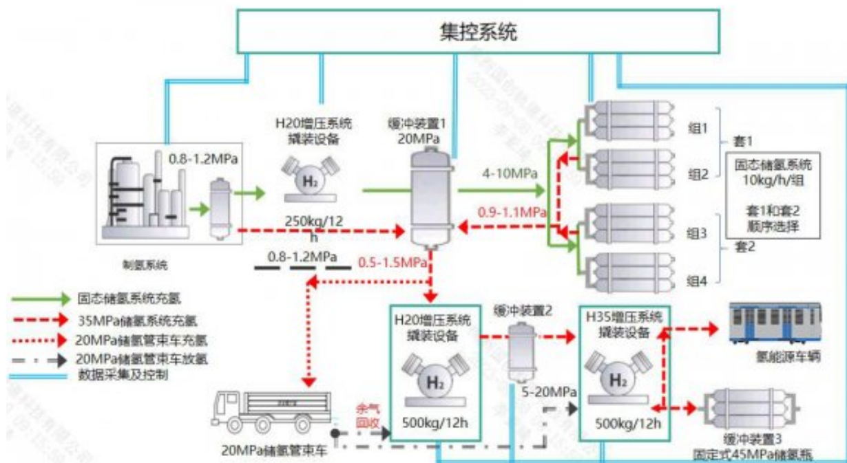
图11 工艺装备布置图
