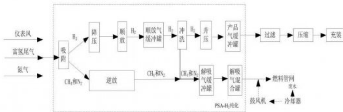
图15 工艺路线图
