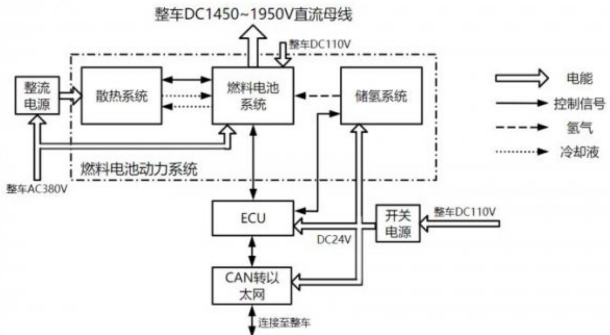
图4 燃料电池动力系统拓扑图
