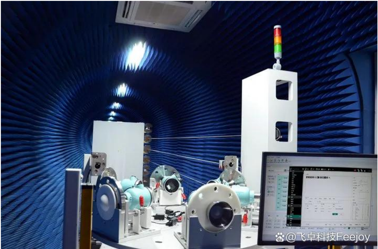
雷达标定线
