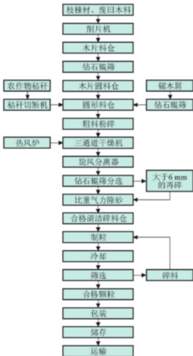
图2 生物质颗粒燃料生产工艺流程图
