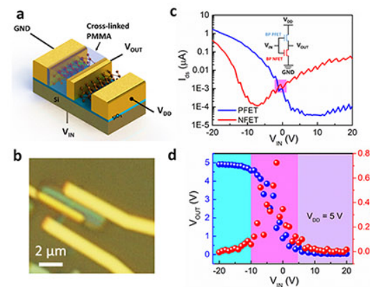
图4. (a) 黑磷逻辑反相器的器件示意图。(b) 器件的光学显微镜图片。(c) 器件中分立n和p-型场效应晶体的转移特性曲线。(d) 逻辑反相器的输出信号及增益与输入信号间的变化曲线。
