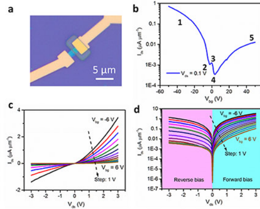
图2. (a) 黑磷二极管的光学显微镜图片。(b) 器件的转移特性曲线。(c) 线性坐标系下, 在不同背栅电压调控下的输出特性曲线, 清晰地显示了其整流作用。(d) 对数坐标系下, 在不同背栅电压调控下的输出特性曲线。
