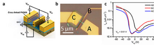
图1. (a) 覆盖过厚PMMA的黑磷器件与单纯黑磷器件串联结构示意图。(b) 相应器件光学显微镜图片。(c) 图(b)中所示电极的对应器件的转移特性曲线。
