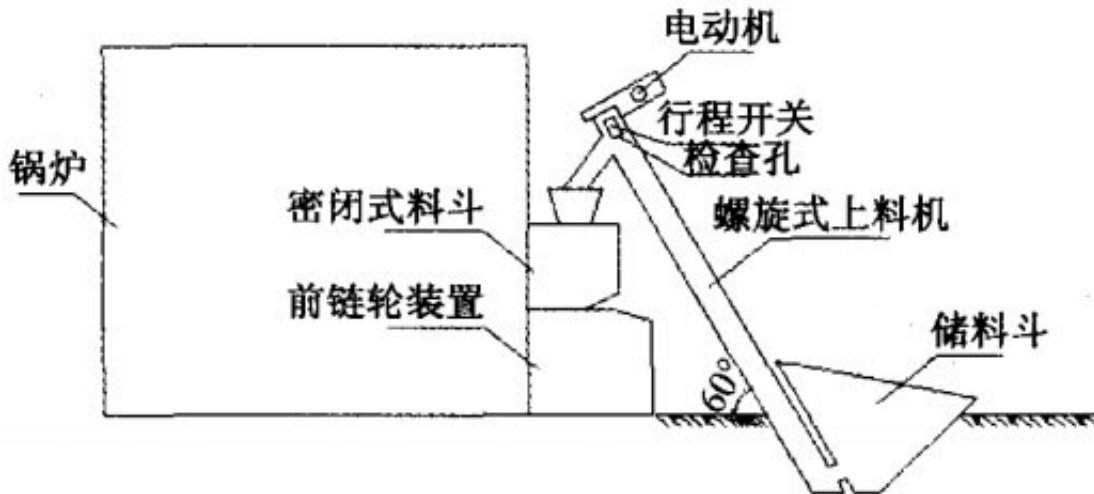
图 1 螺旋式上料机安装示意图
