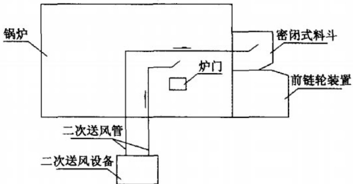
图 2 二次送风设备安装示意图
