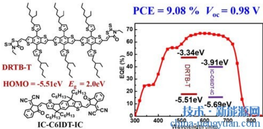
非富勒烯全小分子太阳能电池材料与性能示意图
