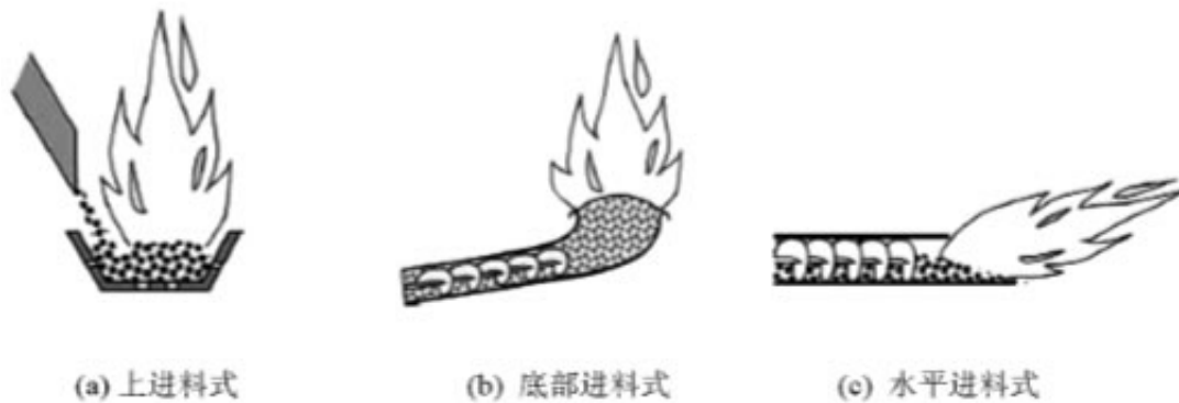
图1 燃烧器的三种进料形式 [20]
