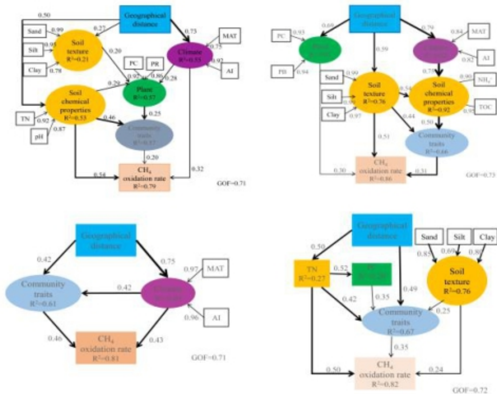
不同亚区域和区域尺度上影响土壤甲烷氧化潜势的路径模型分析
