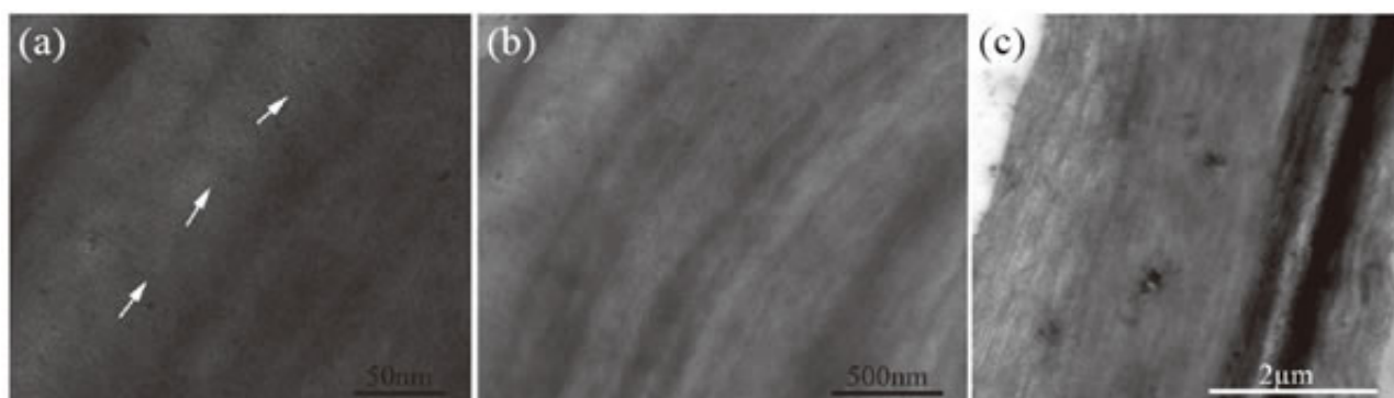
图 2 超微结构的细胞化学染色定位木质素在细胞壁中的位置图 [8]
