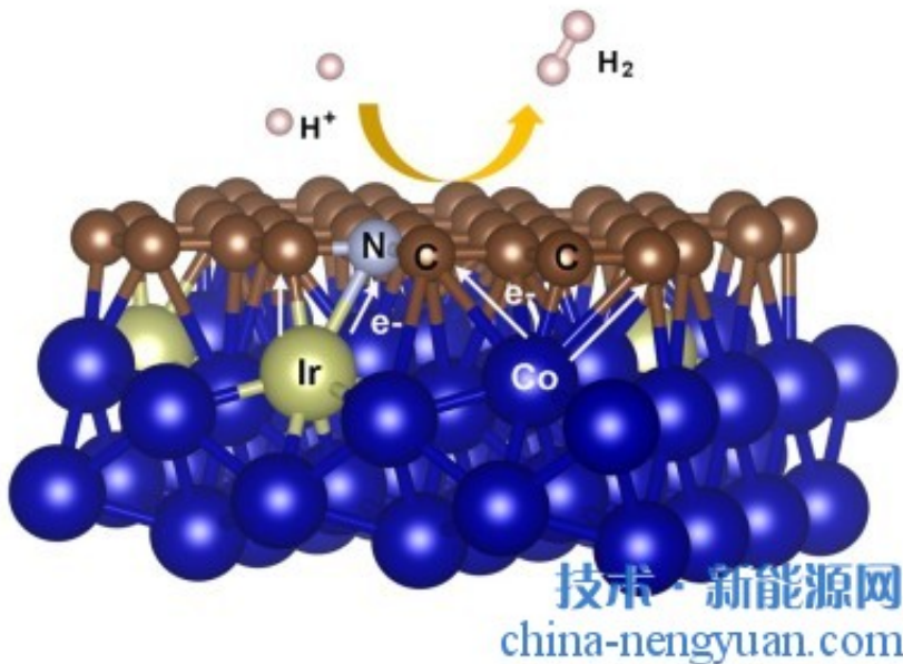
催化剂结构及电催化析氢反应示意图
