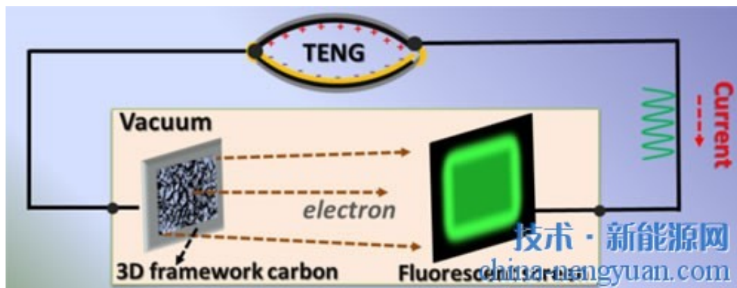
TENG驱动3D网络碳冷阴极示意图
