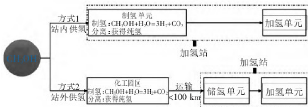
图2 甲醇制氢的应用方式
