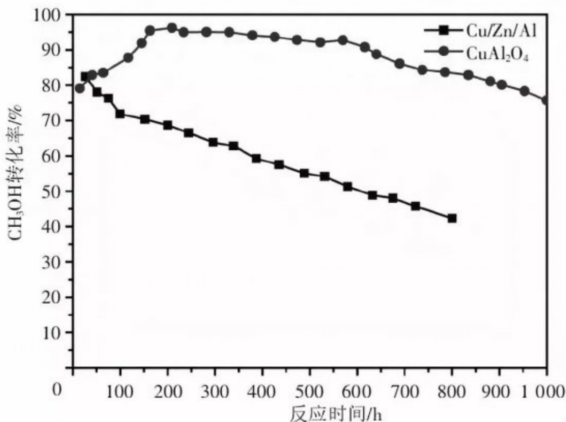
图1 CH 3 OH 转化率随反应时间的变化
