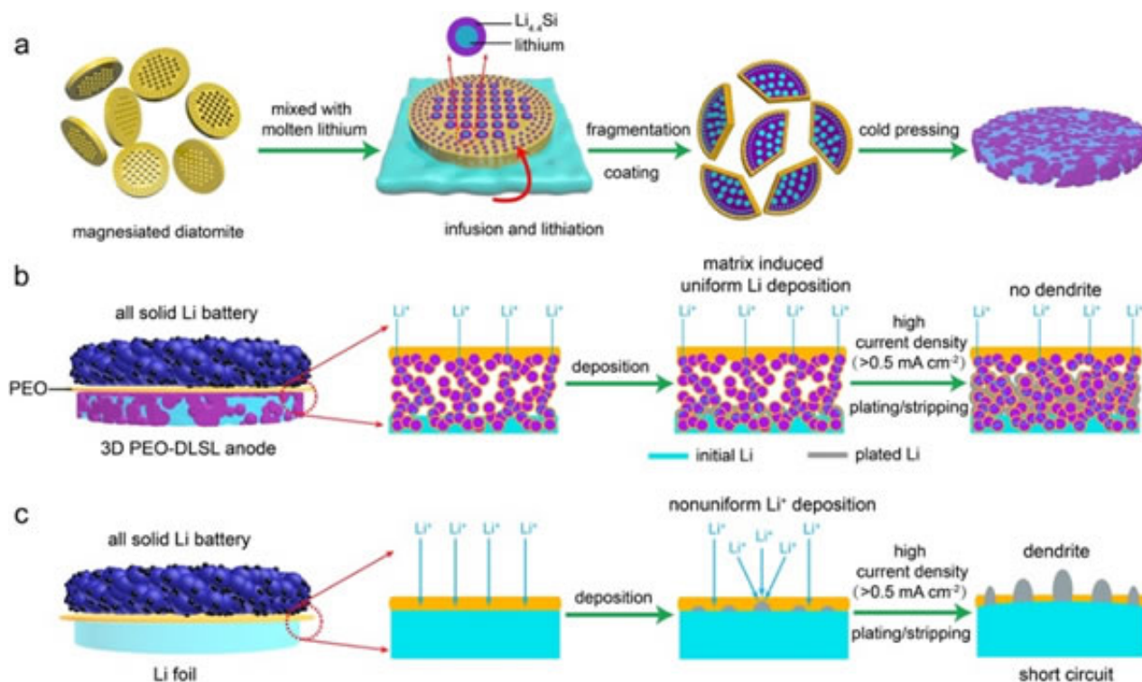
图1: (a) 硅藻土模板衍生的多级结构固态锂金属复合负极的制备过程示意图。(b) 多级结构固态锂金属复合负极的锂沉积/脱出示意图。(c) 平板锂箔负极的锂沉积/脱出示意图。
