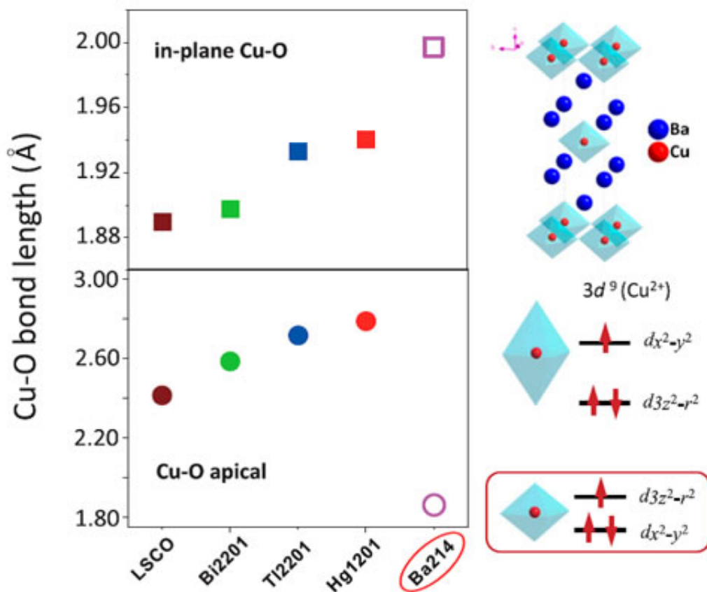
图1. 具有单层铜氧面结构的铜基超导材料的面内氧和顶角氧的铜氧键长、铜氧配位构型、铜的 3d_{x^2-y^2} 和 3d_{z^2-r^2} 轨道相对顺序。其中La系、Bi系、Tl(Hg)系的顶角氧距离大于面内铜氧键长, 呈现拉伸型铜氧六配位构型, 导致 3d_{x^2-y^2} 轨道居于 3d_{z^2-r^2} 轨道之上。Ba214的面内铜氧键长大于顶角氧距离, 形成目前唯一的压缩型铜氧配位构型, 导致 3d_{z^2-r^2} 轨道居于 3d_{x^2-y^2} 轨道之上。
