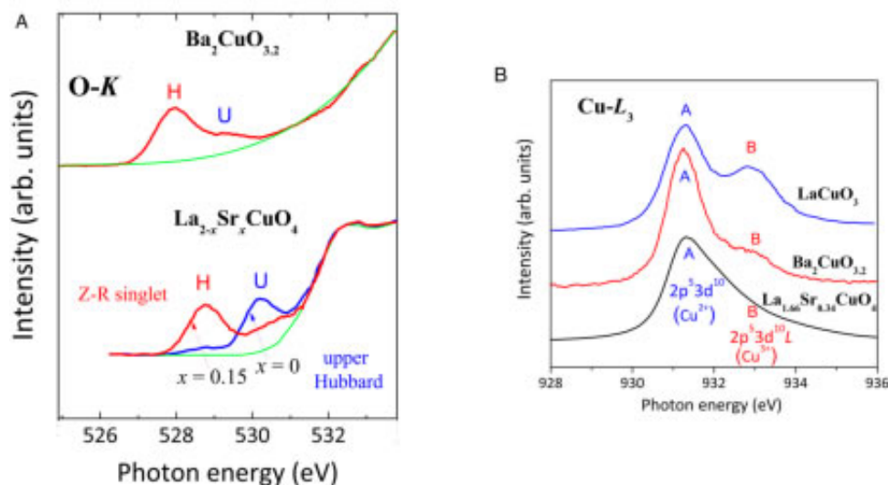
图2. 通过X射线吸收谱测得掺杂浓度。(A) Ba214 and LSCO[x = 0 (blue) and 0.15 (red)]的氧K边吸收谱, U和H分别源于O1s芯能级至铜的上Hubbard带和掺杂空穴态, 对应于Cu 2+ 态和Cu 3+ 态(即Zhang Rice单态)。(B) Ba2CuO3.2、过掺杂的LSCO(x = 0.34)和LaCuO3的铜L边吸收谱, 表明Ba2CuO3.2铜的价态处于超过掺杂状态。
