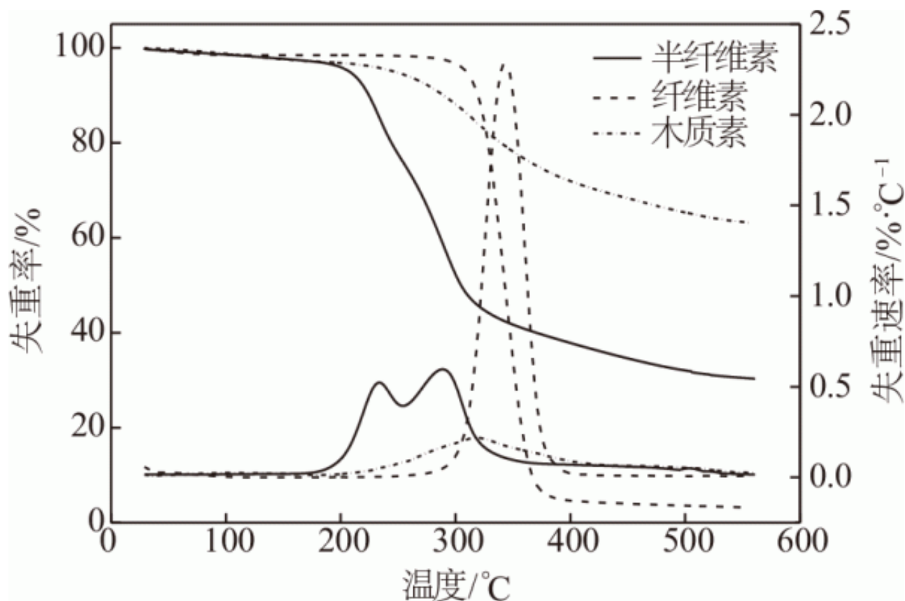
图1 单组分的TG-DTG曲线
