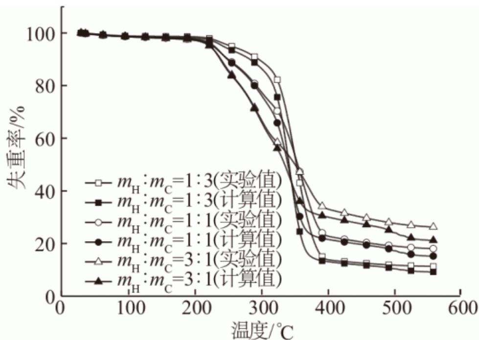
a. TG 曲线
