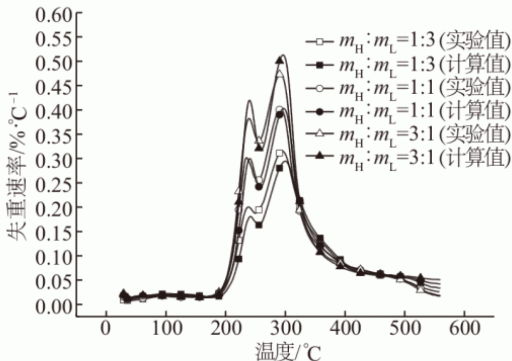
b. DTG 曲线
