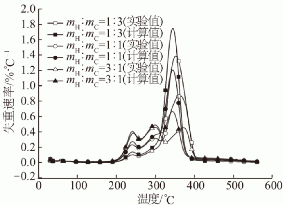
b. DTG 曲线
