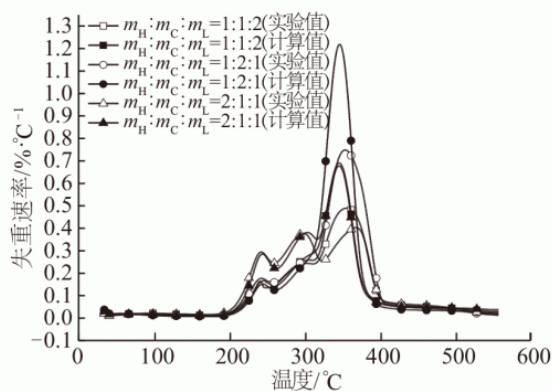
b. DTG 曲线
