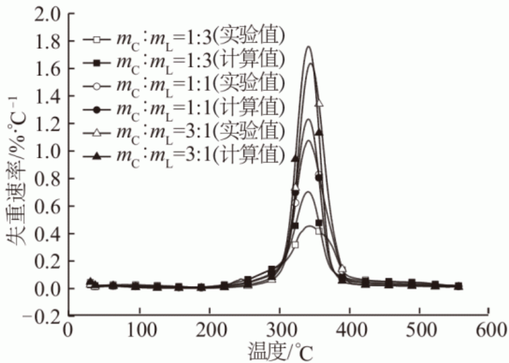
b. DTG 曲线
