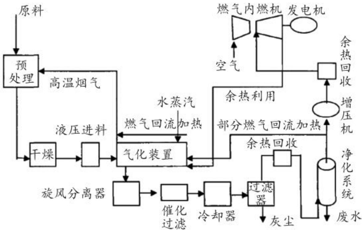
图3 生物质-垃圾水蒸汽全气化系统流程
