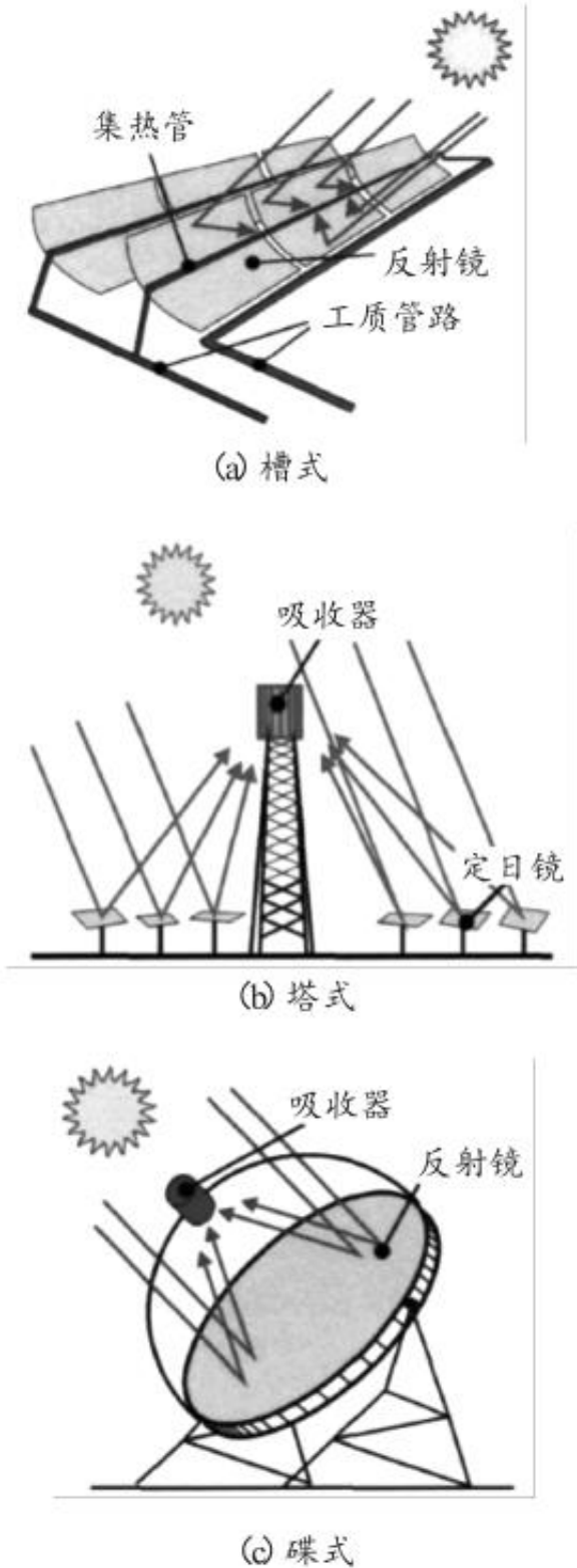
图1 太阳能发电集热装置
