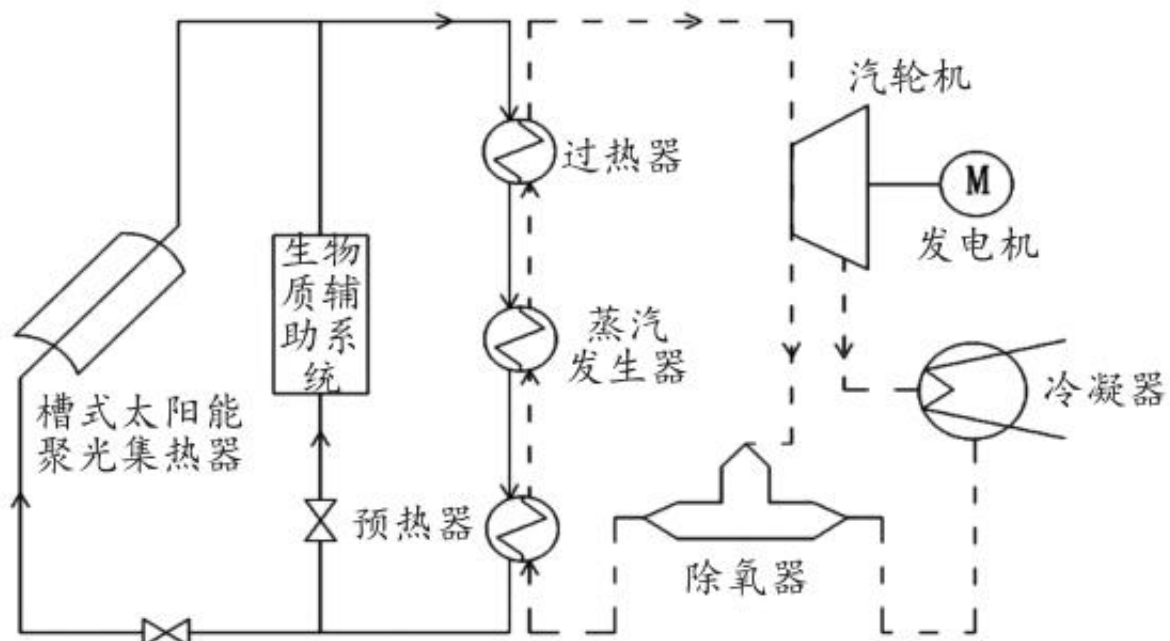
图2 生物质能和太阳能联合发电系统
