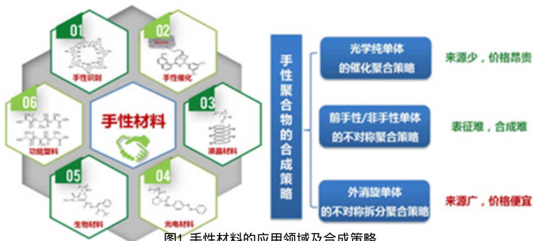
图1. 手性材料的应用领域及合成策略
