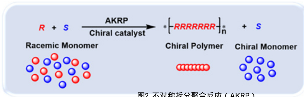
图2. 不对称拆分聚合反应 (AKRP)
