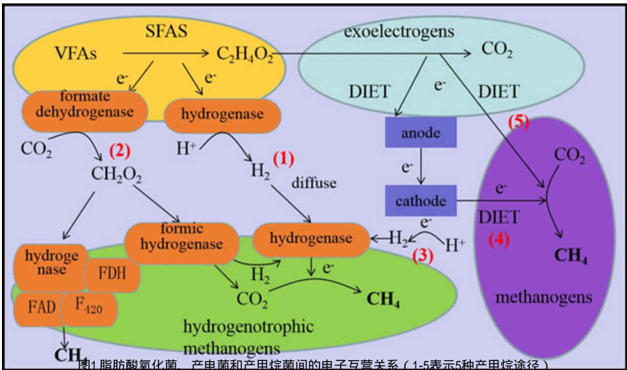
图1 脂肪酸氧化菌、产电菌和产甲烷菌间的电子互营关系（1-5表示5种产甲烷途径）
