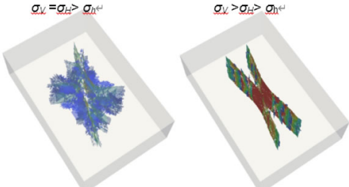
图3.含天然裂缝岩体中地应力对水力压裂改造形成的三维裂缝网络形态的影响
