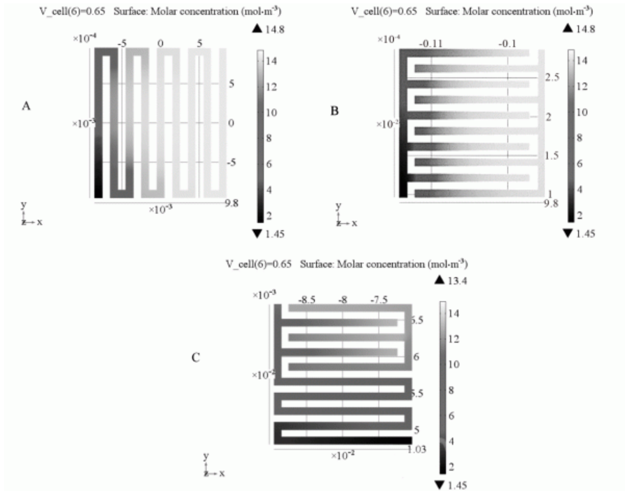
图 4 三种流道下的阴极水浓度
