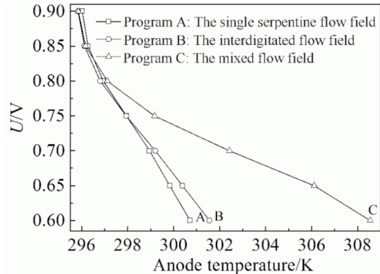
图 6 阳极温度变化
