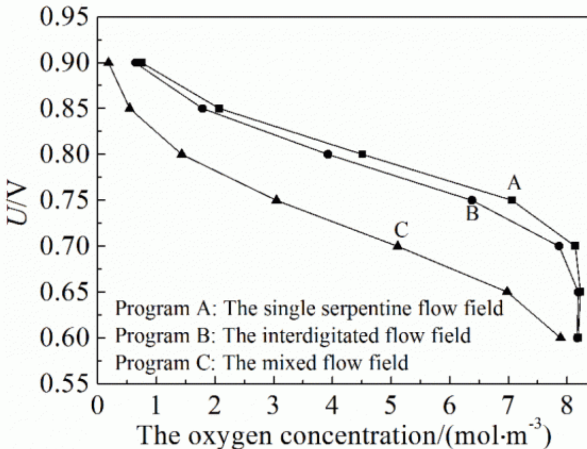
图 3 三种流道的进出口氧气浓度差
