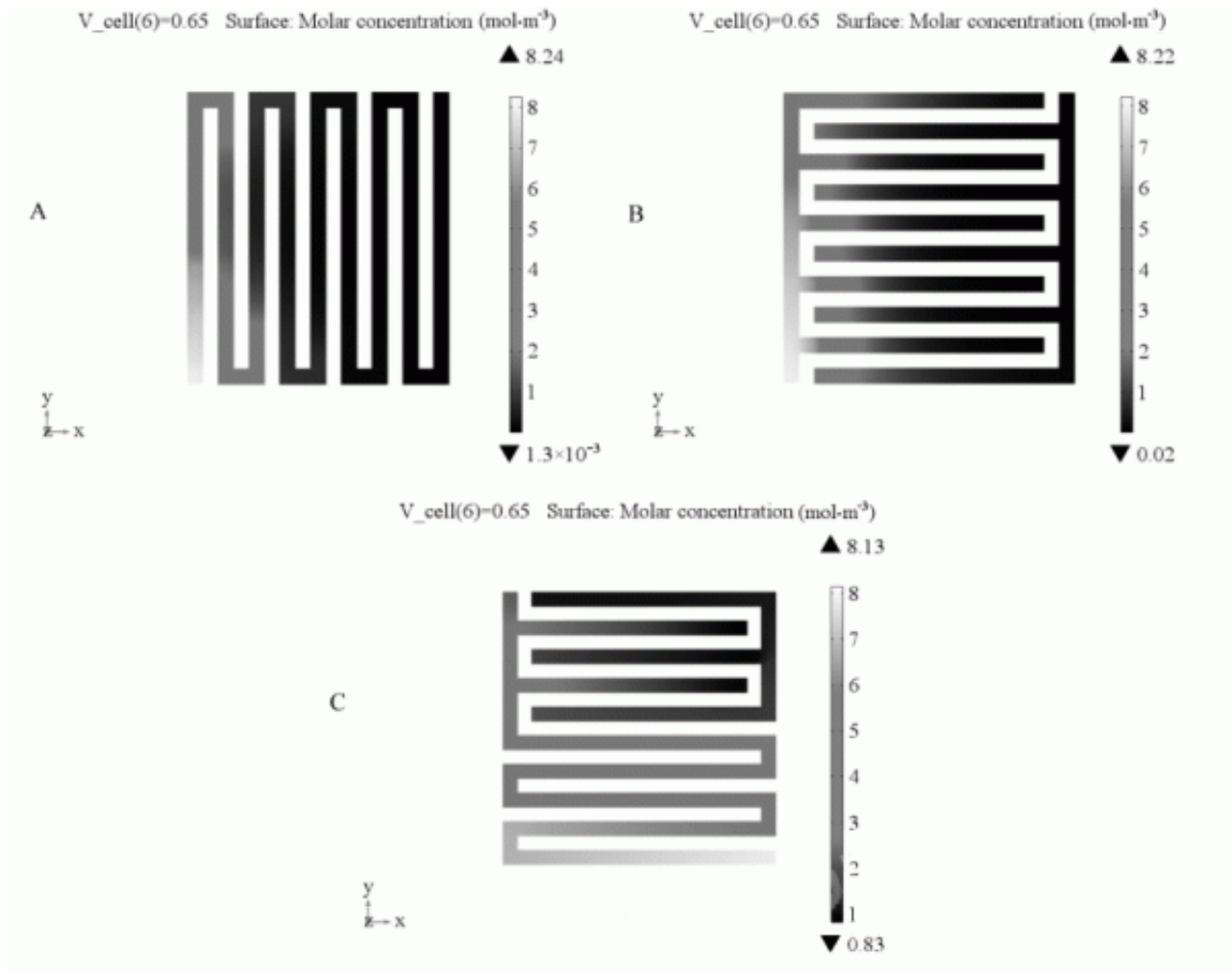
图2 三种流道下的阴极氧气浓度分布
