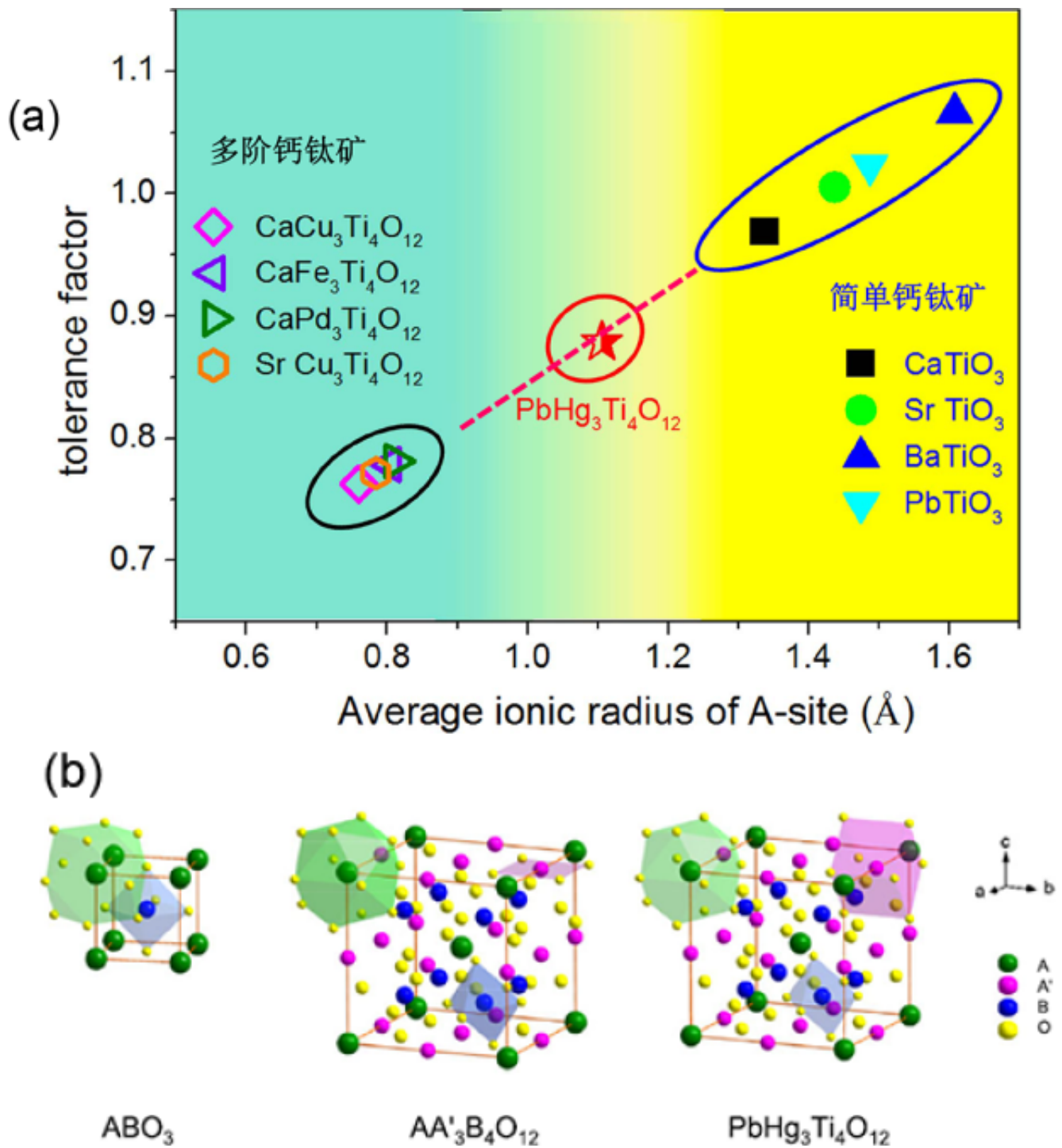
图1.简单钙钛矿和A位有序四阶钙钛矿 (a) A位离子平均半径和容忍因子之间的对应关系；简单钙钛矿、A位有序普通四阶钙钛矿、PHTO四阶钙钛矿的配位结构
