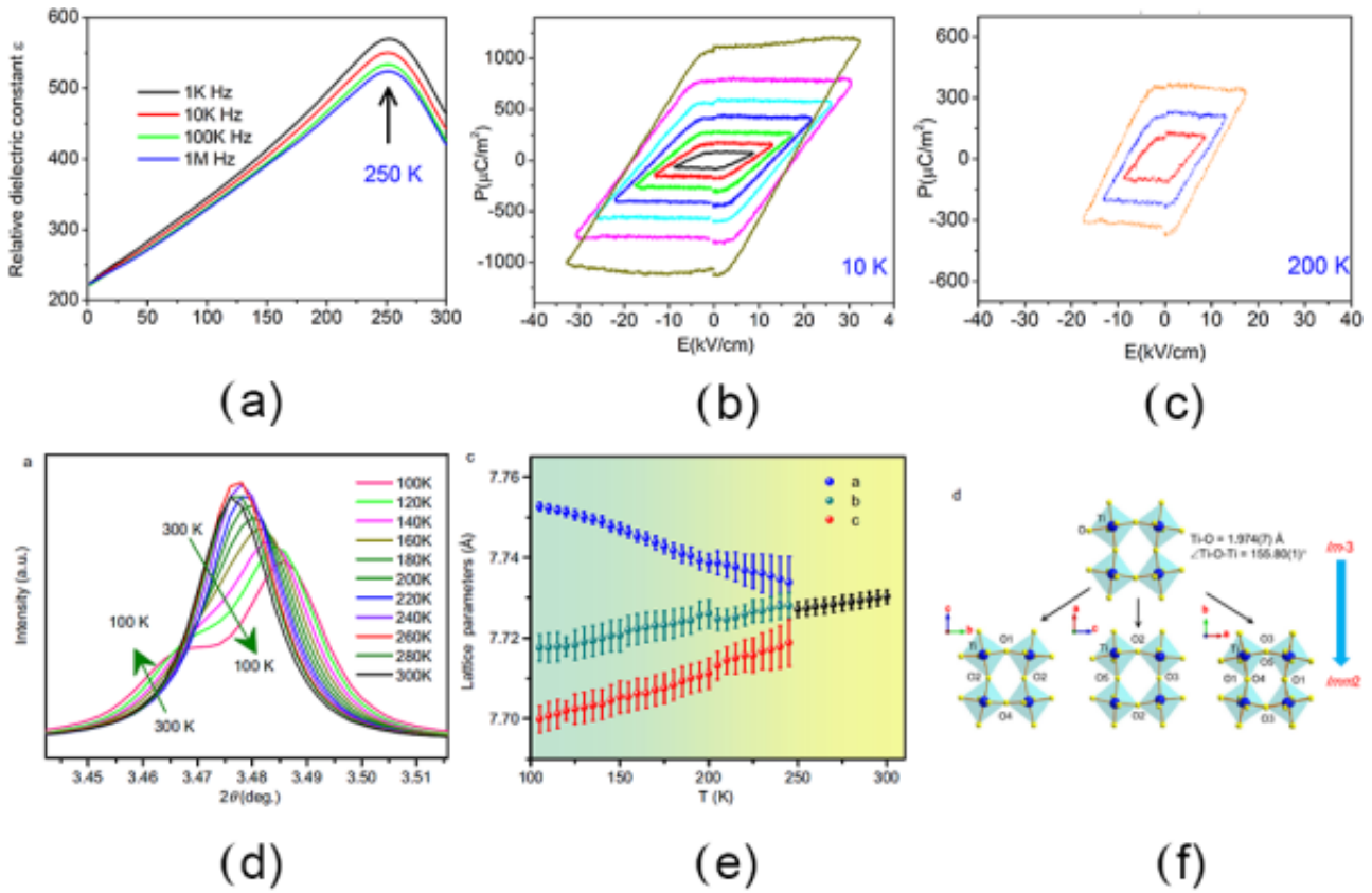
图2.PHTO介电和铁电性能 (a~c) ; 特征衍射峰、衍射谱、晶格常数随温度的变化和TiO 6 八面体在结构相变前后变化的示意图 (d~f)
