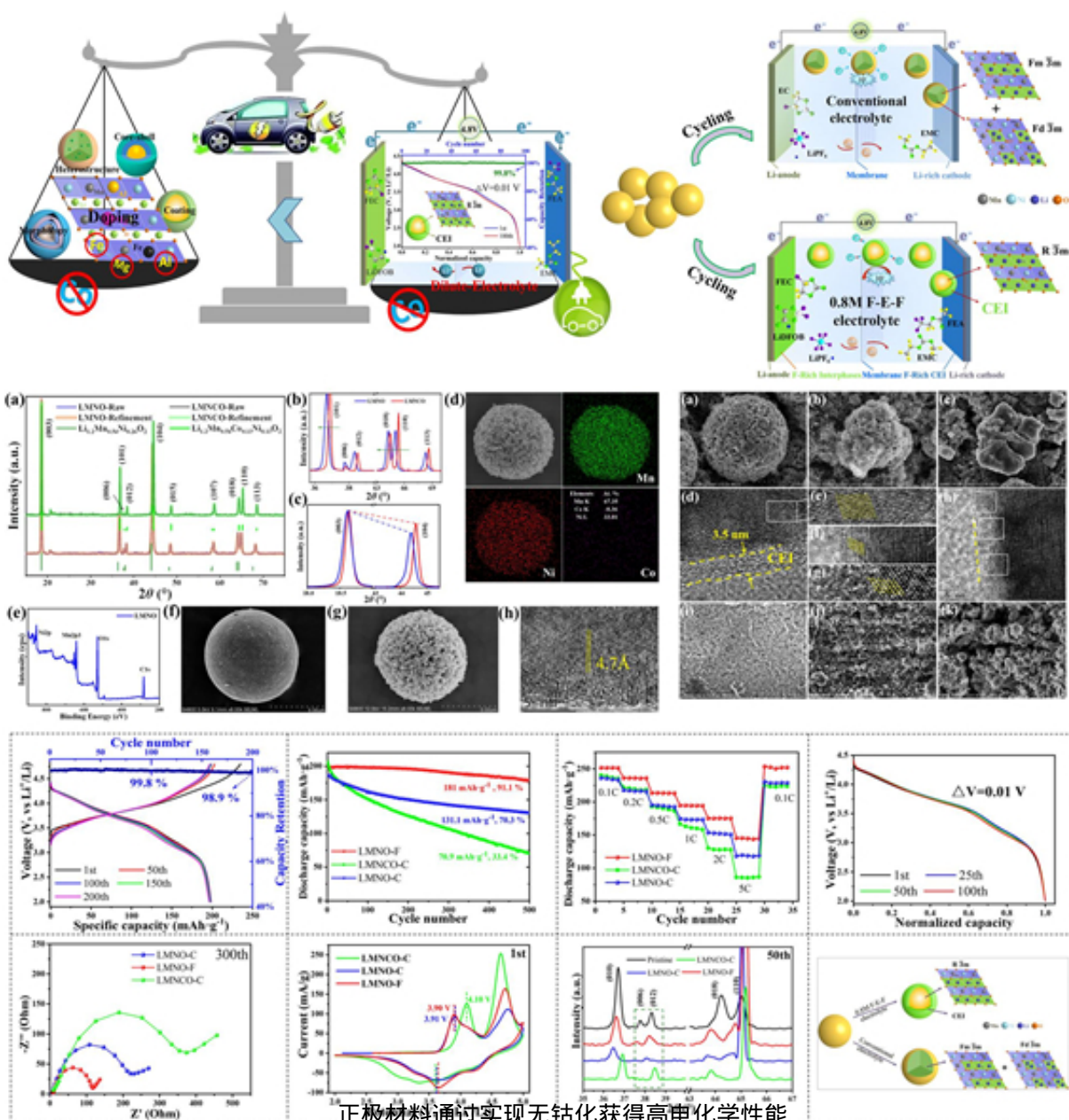
正极材料通过实现无钴化获得高电化学性能
