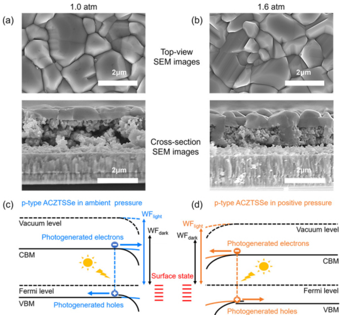
图2. (a) 对比组吸收层的SEM正面和截面图像；(b) 实验组吸收层的SEM正面和截面图像；(c) 对比组吸收层的能带结构；(d) 实验组吸收层的能带结构。
