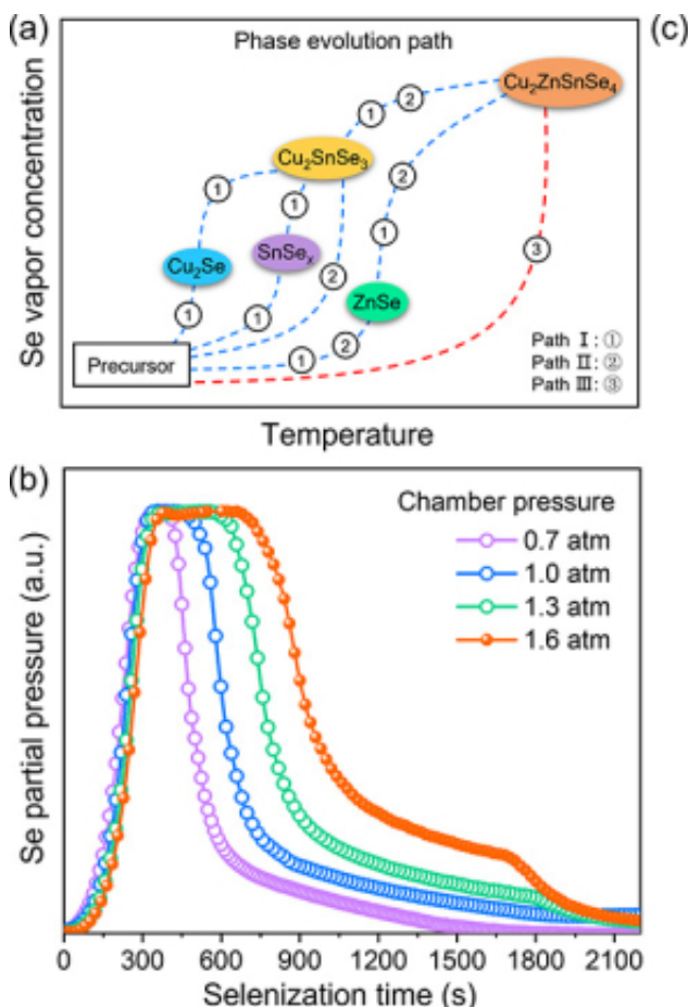
图1. (a) 铜锌锡硫硒的相演变路径示意图；(b) 原位监测获得的不同腔压下反应过程中的硒分压曲线；(c) 铜锌锡硫硒太阳能电池认证报告（国家光伏产业计量测试中心）。
