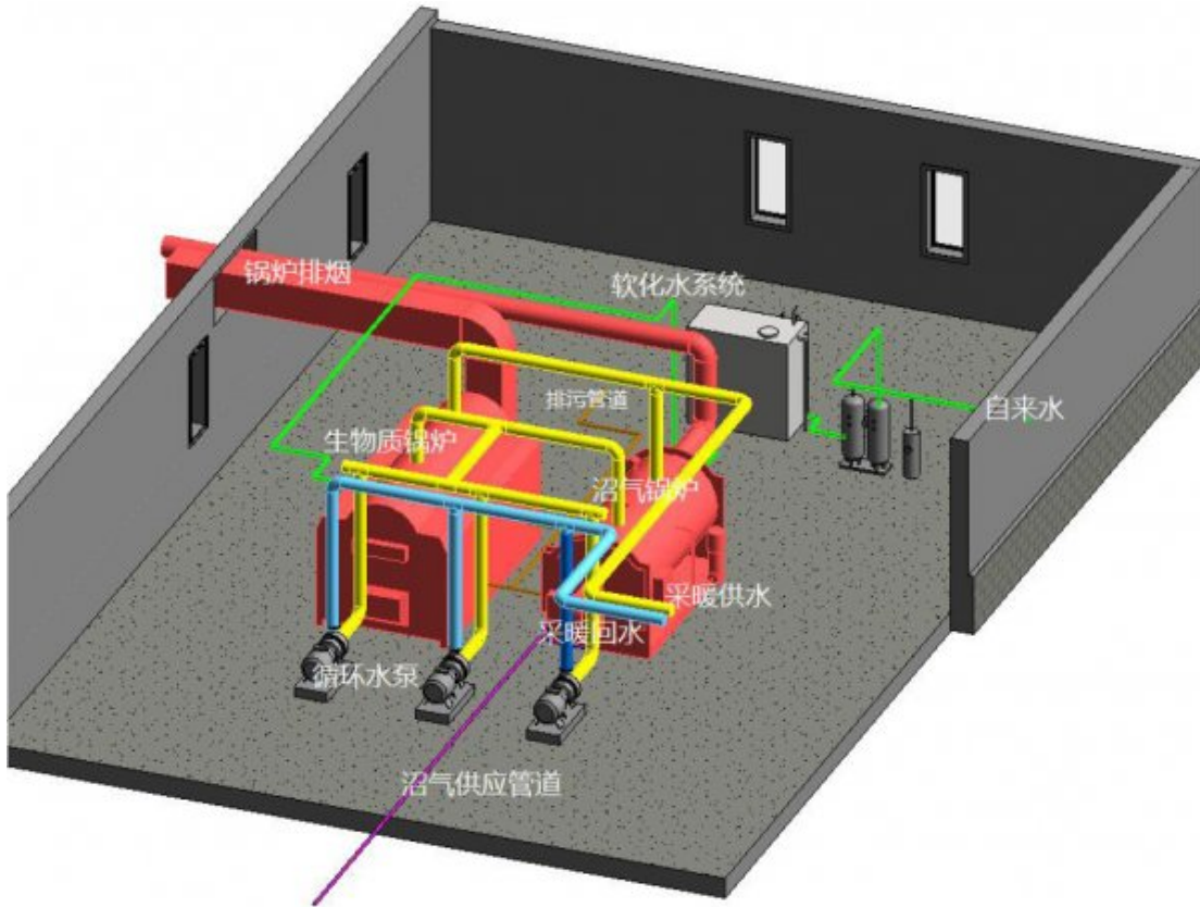
a. 村能源站供热锅炉房配置
