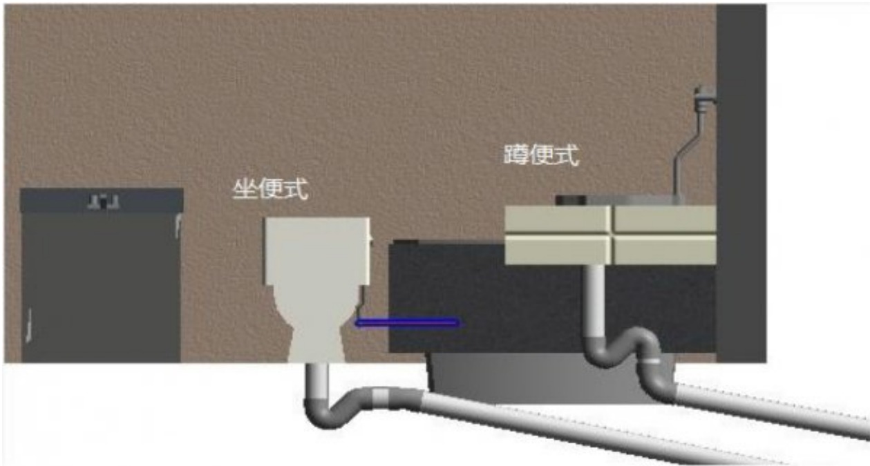
a. 厕所排水管示意图
