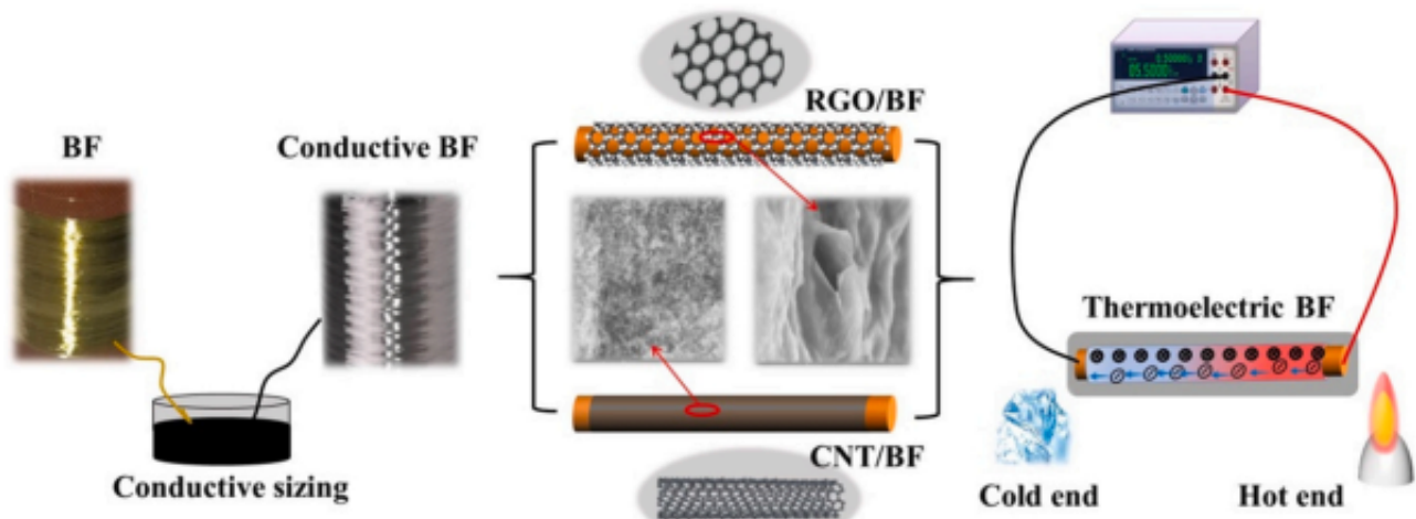
玄武岩纤维基热电转换材料的制备及工作原理
