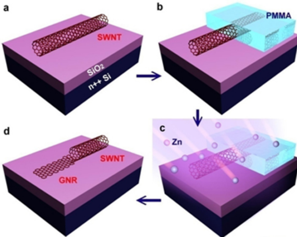
单壁碳纳米管/石墨烯带分子内结的制备过程
