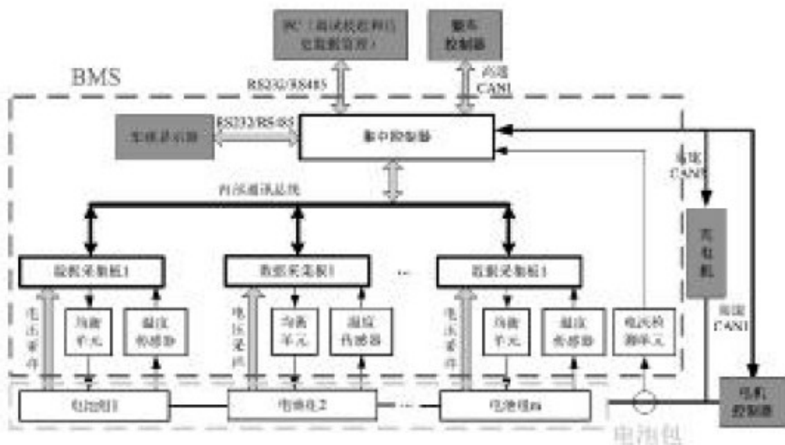
图1 电池管理系统框图
