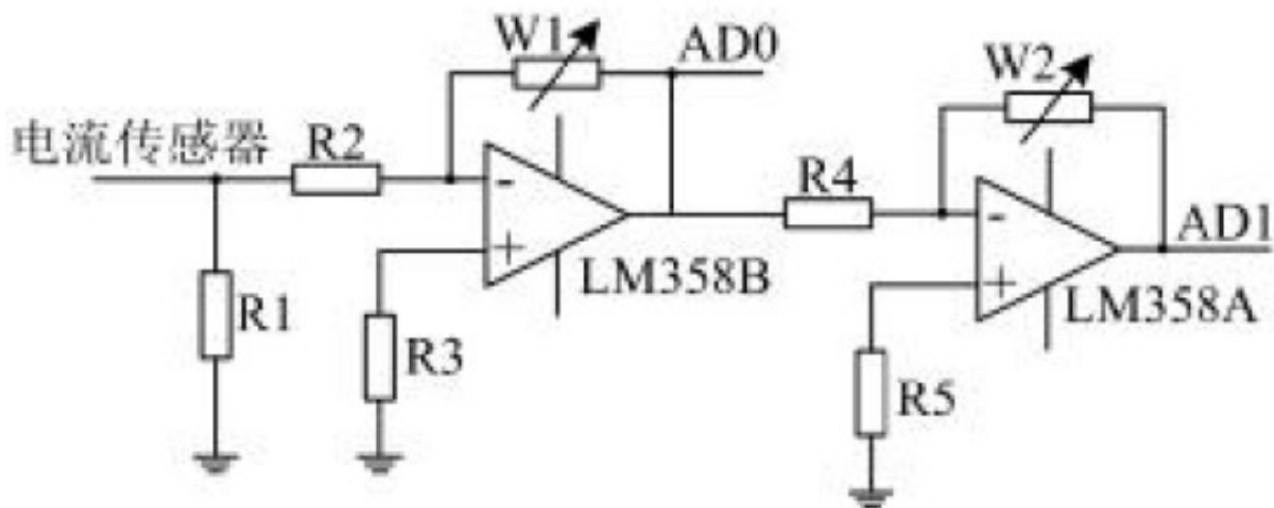
图3 电流采样原理图
