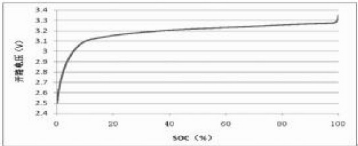
图4 SOC开路电压曲线
