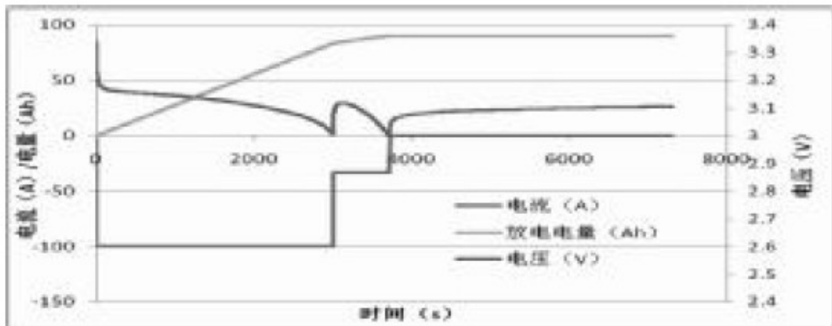
图5 放电曲线
