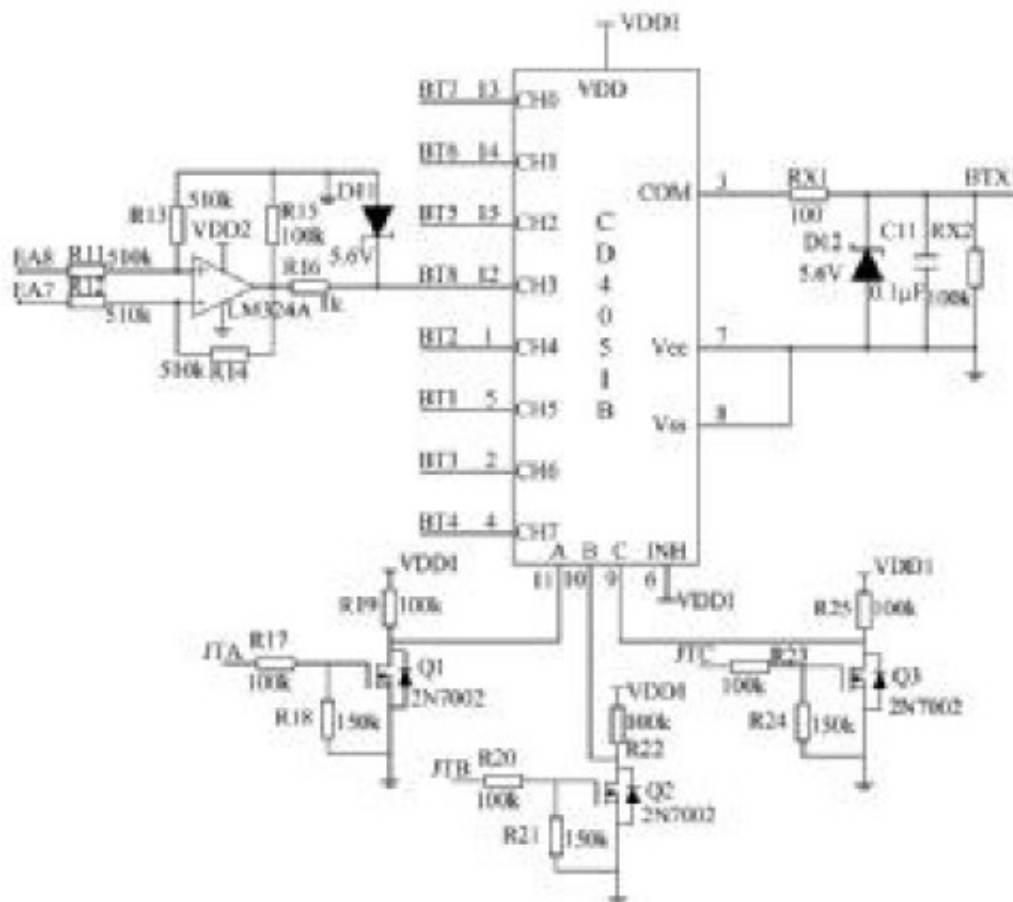
图2 电压采集电路
