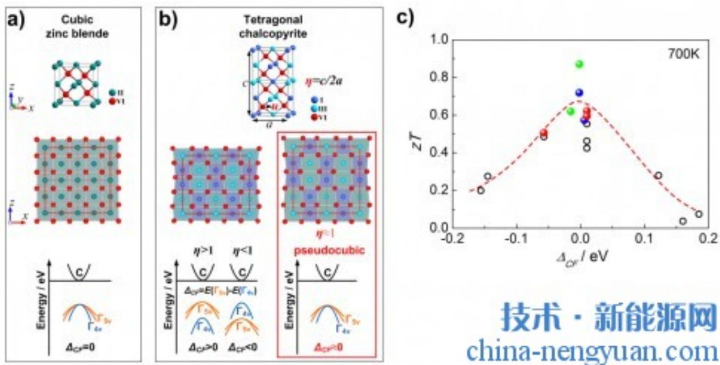
图1 在非立方黄铜矿结构化合物中，“赝立方”结构设计方法实现类似于立方结构的高度简并能带，从而得到良好的电输运性能和热电性能。（a）立方闪锌矿结构的晶体结构和能带结构示意图。（b）三元黄铜矿结构化合物的晶体结构和能带结构示意图。“赝立方”结构由一个立方的阳离子框架和非立方扭曲的阴离子网格组成。（c）ZT值随价带顶能带劈裂值 \Delta_{CF} 的变化关系。红色的点代表已报道的高温 ZT>1 的化合物，蓝色和绿色的点分别代表 (Ag,Cu)InTe_2 和 Cu(In,Ga)Te_2 固溶体。
