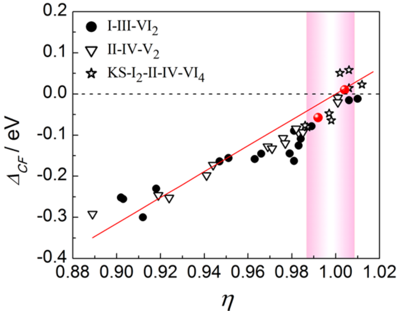
图2 Unity- \eta 筛选准则。红色的点代表已报道的高温 ZT > 1 的化合物。粉色彩带标出 \eta \approx 1 区域（性能良好的热电化合物可能存在的区域）。
