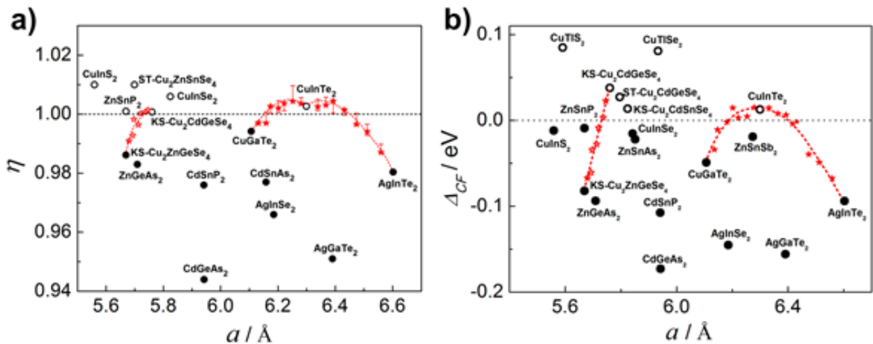
图3 (a) \eta vs. a 和(b) \Delta_{CF} vs. a 固溶化合物设计图，其中红色的星形代表 \eta < 1 ( \Delta_{CF} < 0 )和 \eta > 1 ( \Delta_{CF} > 0 )的两种化合物形成的固溶体，红色虚线是趋势线。
