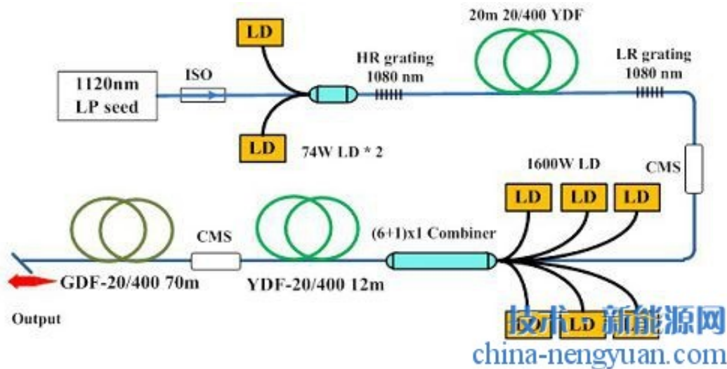
千瓦级掺镱-拉曼集成的光纤放大器结构示意图
