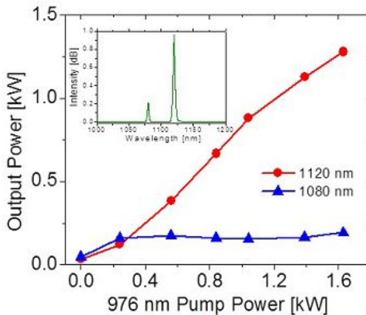
输出功率随976 nm二极管泵浦功率的变化曲线，其中的插图为最高输出时的光谱。
