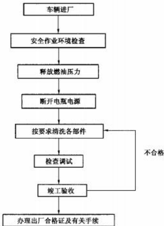
图 1 清洗工艺流程
