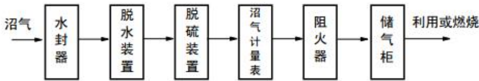
图5 沼气净化系统图
