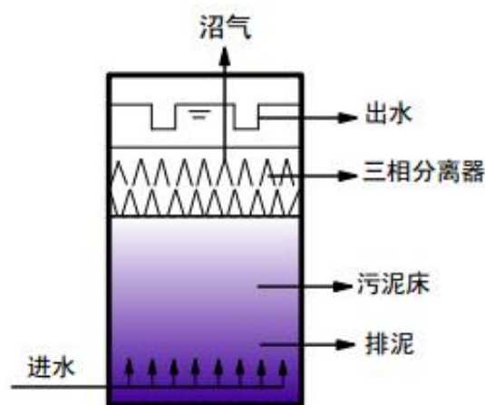
图 3 UASB 反应器结构示意图
