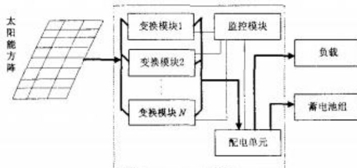
图2 输入并联型控制器系统原理
