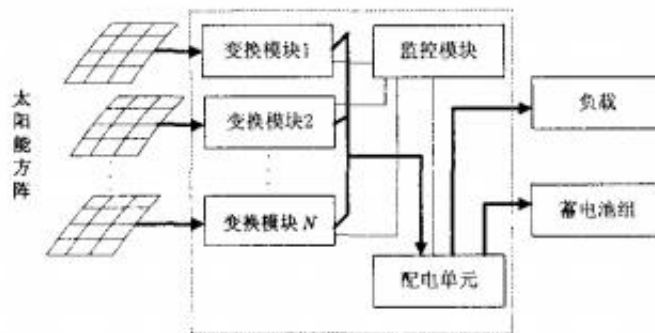
图1 非输入并联型控制器系统原理
