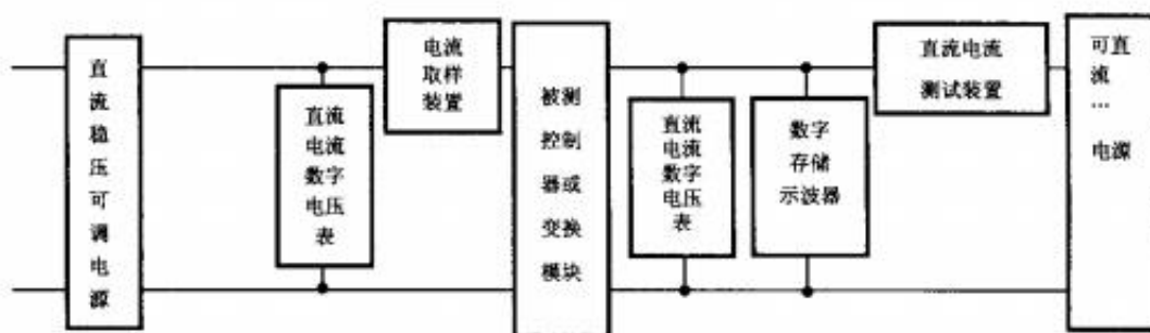
图3-2 试验基本原理
