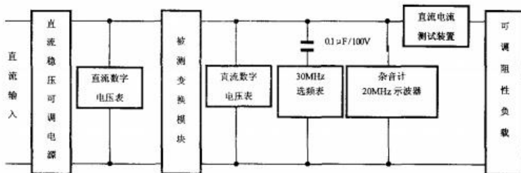
图5 杂音电压试验电路
