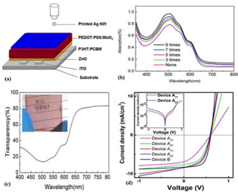
图2. (a) 所采用的OPV器件结构和喷墨打印示意图；(b) 打印不同遍数银纳米线之后的器件吸收测试结果；(c) 采用打印顶部电极的半透明OPV器件在可见光波段的透过率曲线。插图为器件照片，显示半透明效果良好；(d) 典型的器件电流密度-电压 ( J-V ) 曲线，其中器件A 3T 、A 5T 、A 7T 、A 9T 为同一个器件在打印3、5、7、9次电极后的性能对比，器件B为采用真空沉积非透明银电极的参比器件。插图为表现最好的A 7T 与参比器件B的对数电流对比，显示打印电极的整流比有所降低。
