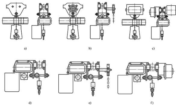
图 2 单轨运行小车式防爆环链电动葫芦
