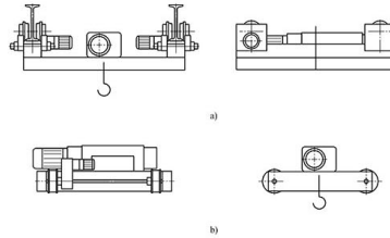
图7 双梁小车式防爆钢丝绳电动葫芦
