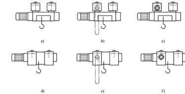
图5 直线单轨运行小车式防爆钢丝绳电动葫芦
