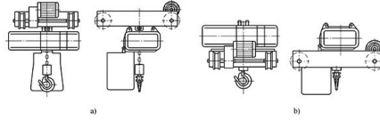
图3 双梁小车式防爆环链电动葫芦
