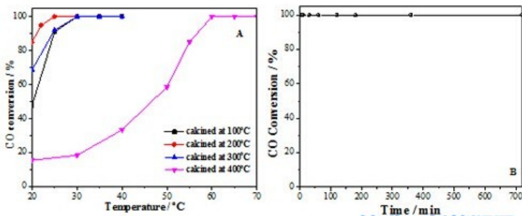
不同焙烧温度催化剂的活性(A)及最优催化剂的热稳定性(B)
