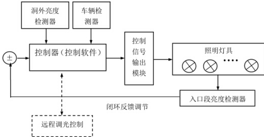
图1 控制系统构成图
